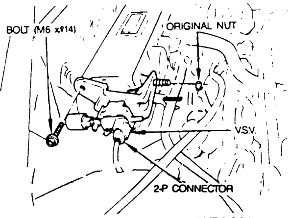
FX-16 (P/N 90081-91002) VSV
